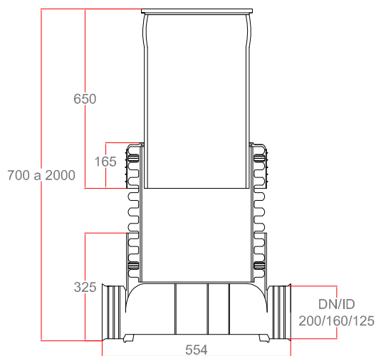
Vista seccionada del conjunto
